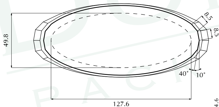
Détail bague / Finish Echelle / Scale 1:1
