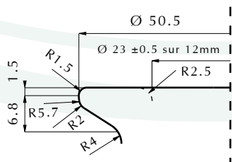
Détail bague / Finish Echelle / Scale 1:1
